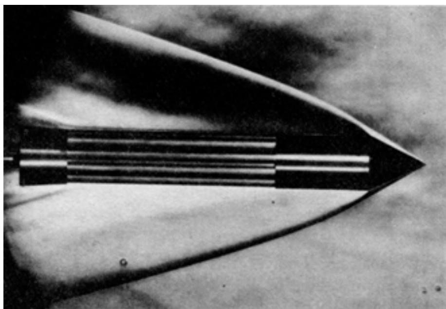
图 51.2: 超音速抛射体在气体中所产生的冲击波
