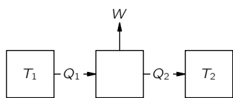
图 44.3: 热机
