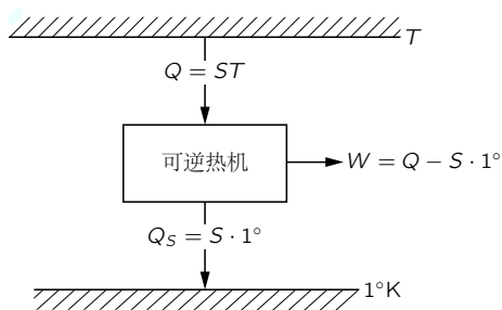
图 44.9: 绝对热力学温度
