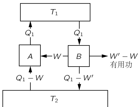
图 44.7: 热机 B 使可逆机 A 反向运转
