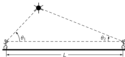
图 5.4: 用三角法测定人造卫星的高度
