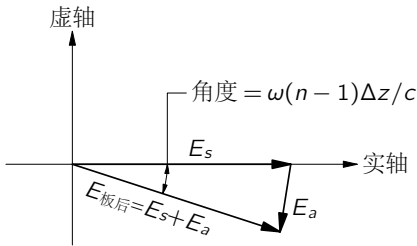
图 31.3: 在某一特定的 t 和 z 时的透射波复矢量图
