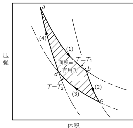
图 44.6: 卡诺循环
