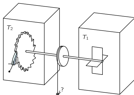
图 46.1: 棘轮和掣爪机械
