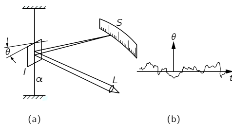
图 41.1: (a) 光束式灵敏电流计，来自光源 L 的光束经小镜反射后射至刻度尺上；(b) 刻度的读数作为时间的函数的记录图
