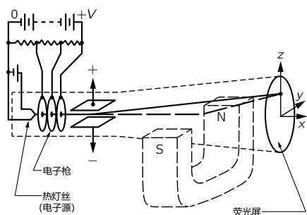
图 12.3: 电子束管
