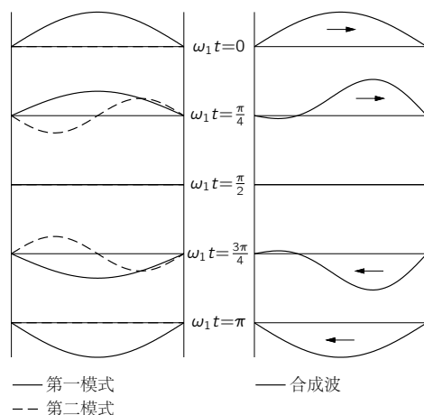
图 49.3: 两种模式组合成一个行波
