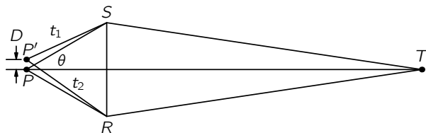
图 27.9: 光学系统的分辨本领
