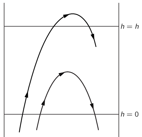
图 40.4: 只有那些具有足够速度的分子从 h = 0 向上移动才能够到达 h 的高度
