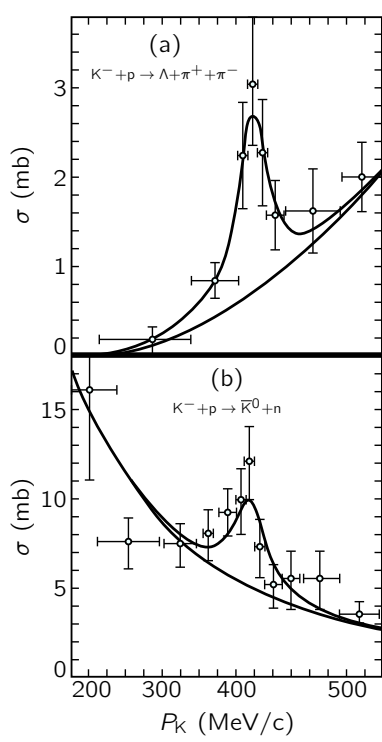
图 23.10: 动量与反应截面的依赖关系 (a) K^- + p \rightarrow \Lambda + \pi^+ + \pi^- 和 (b) K^- + p \rightarrow \bar{K}^0 + n 。在 (a) 和 (b) 中下面的曲线代表假定的非共振背景，而上面的曲线是在背景上再叠加共振。 (转载自 Ferro-Luzzi M, et al. Phys Rev Lett, 1962, 8:28)
