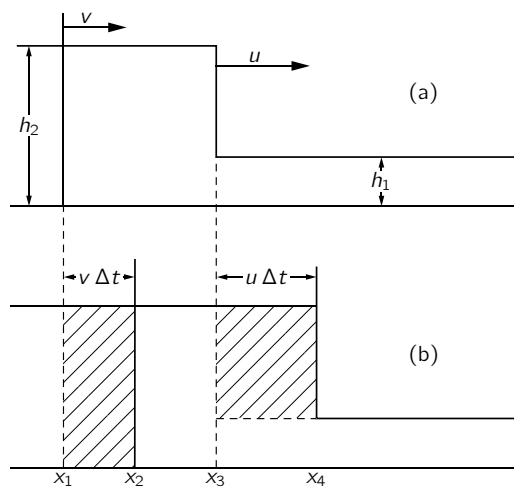
图 51.5: 水槽中一个激浪的两个横截面，其中 (b) 比 (a) 迟
