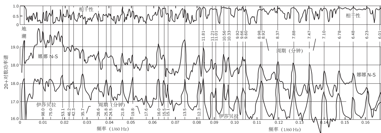
图 51.7: 在秘鲁的娜娜 (Ñaña) 和加利福尼亚的伊莎贝拉 (Isabella) 的地震仪上所探测到的功率与频率的函数关系。图中所示的相干性可作为这两个地震台之间的耦合程度的量度
