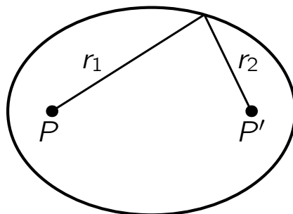
图 26.11: 椭球面镜
