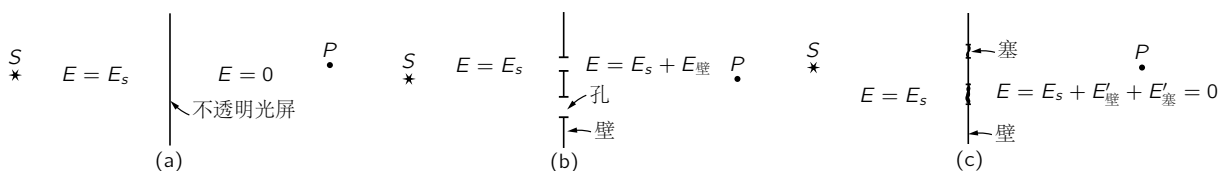
图 31.6: 屏的衍射
