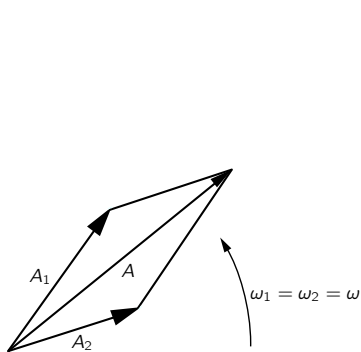
图 48.2: 两个相同频率复矢量的合成
