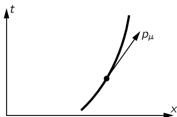
图 17.4: 一个质点的四维动量矢量
