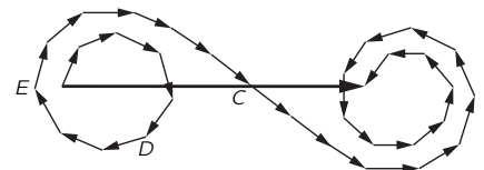
图 26.14: 许多邻近路径的概率振幅总和
