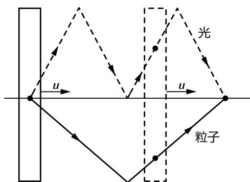
图 16.1: 光和“粒子”在一个运动的钟内的运动轨迹
