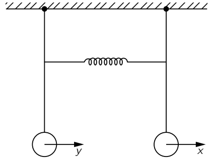
图 49.5: 两个耦合摆
