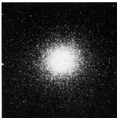
图 7.8: 球状星团
