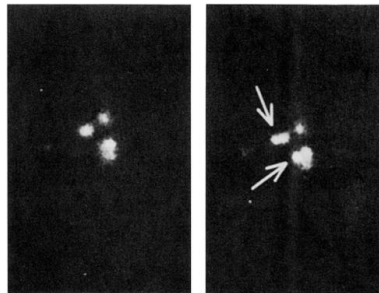
图 7.12: 新星的形成
