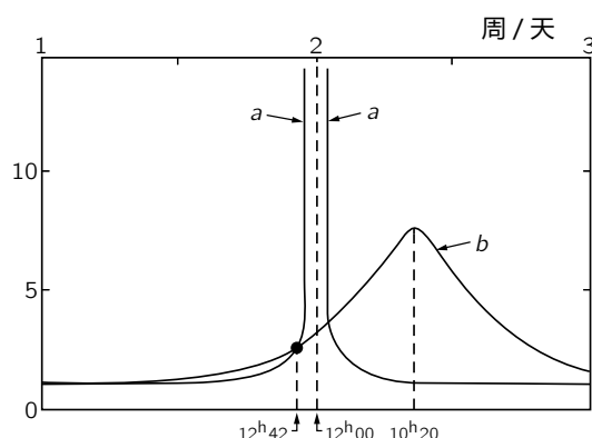
图 23.5: 大气层对外来激发的响应，如果大气层 S_2 —潮汐是由万有引力引起的， a 就是这种条件下所需的响应；峰值的放大率是 100 : 1。 b 是从 M_2 —潮汐观察的倍数和相位导出的。（转载自 Munk W H, MacDonald G J F. Rotation of the Earth. London: Cambridge University Press, 1960）
