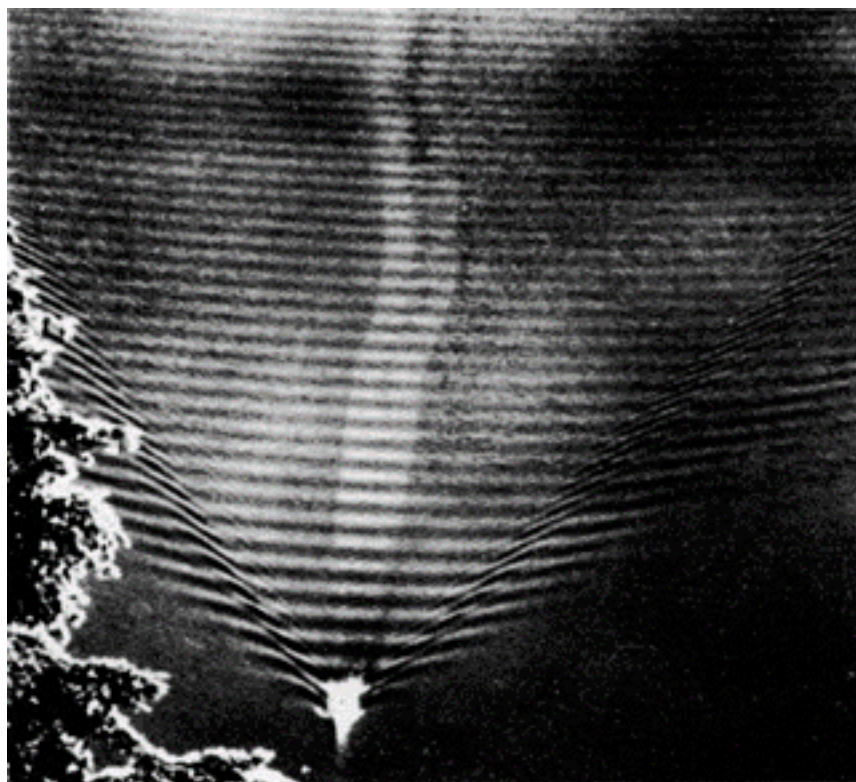
图 51.10: 小船的尾流
