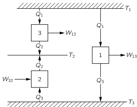
图 44.8: 热机 1 与 2 联合起来等于热机 3
