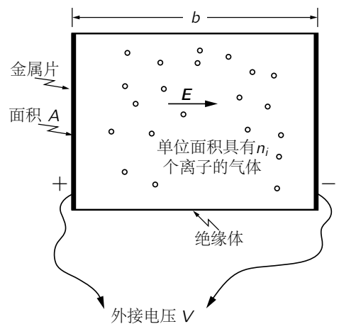
图 43.2: 电离气体的电流
