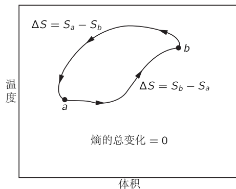
图 44.11: 在完全可逆循环中熵的改变
