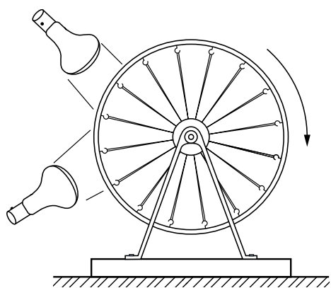
图 44.2: 橡皮带加热机
