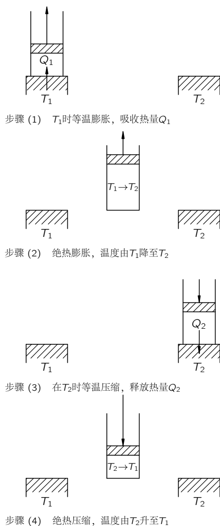
图 44.5: 卡诺循环中的各个步骤
