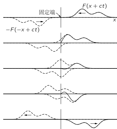
图 49.1: 把波的反射看作为两个行波的叠加
