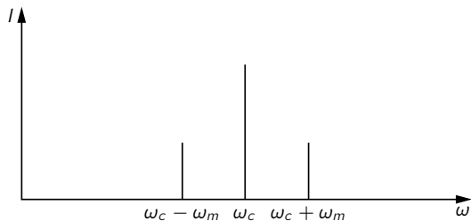
图 48.5: 载波 \omega_c 被单个正弦波 \omega_m 调制时的频谱
