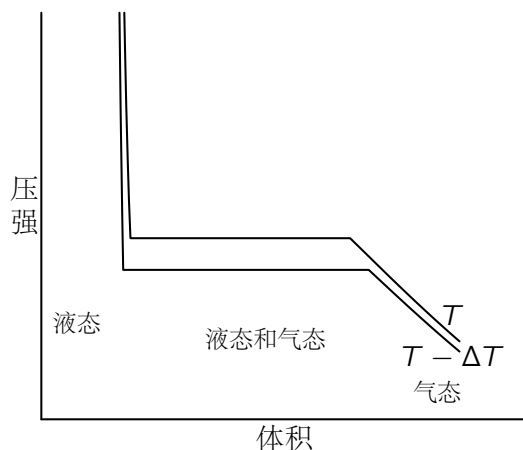
图 45.3: 在汽缸中进行压缩的可凝结蒸气的等温线。在左边,物质处于液相。在右边,物质汽化。在中央部分,液体和蒸气并存
