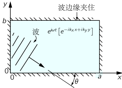
图 49.4: 振动的矩形板
