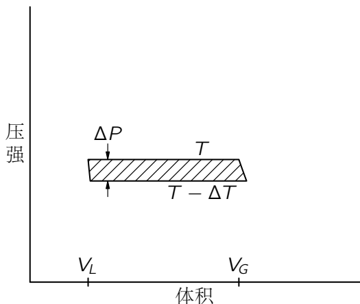
图 45.4: 汽缸中可凝结蒸气的卡诺循环压强-体积图。在左边,物质处于液相。在温度 T 时,加入热量 L 使液体汽化。蒸气绝热膨胀时,温度由 T 变为 T - \Delta T
