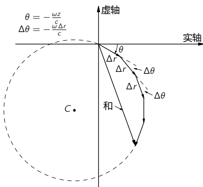
图 30.11: \int_z^\infty e^{-i\omega r/c} dr 的图解
