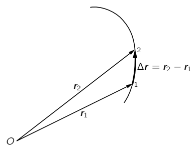
图 11.6: 在短时间间隔 \Delta t = t_2 - t_1 内, 一个粒子的位移
