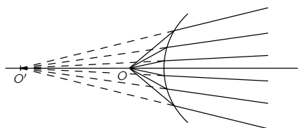
图 27.3: 虚像
