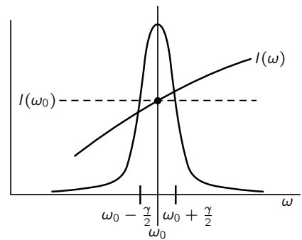
图 41.3: 式 (41.10) 被积函数的因式。图中的峰为谐振曲线 1/[(\omega - \omega_0)^2 + \gamma^2/4] 。作为一个很好的近似，因式 I(\omega) 可用 I(\omega_0) 来代替
