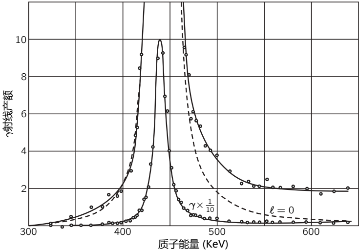
图 23.8: 从 Li 原子中射出的 \gamma 射线强度与轰击质子能量的关系。虚线是对角动量 l = 0 的质子进行计算时得出的理论曲线 (转载自 Bonner T W, Evans J E. Phys Rev, 1948, 73:666)
