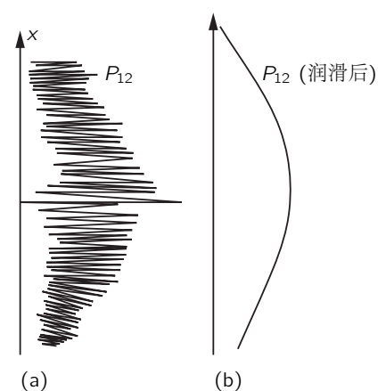
图 37.5: 子弹的干涉实验 (a) 真实的图样（概图）；(b) 观测到的图样
