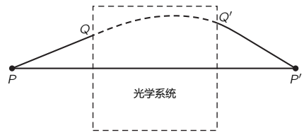
图 26.9: 光学“暗箱”
