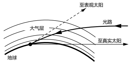
图 26.7: 地平线附件, 表观太阳比真实太阳高出约 1/2 度
