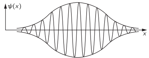
图 48.6: 定域波列
