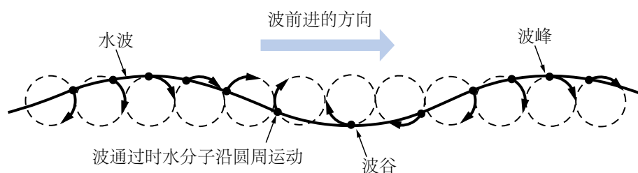
图 51.9: 深水水波是由水的粒子作圆周运动而形成的。注意，圆与圆之间的对称性相移。漂浮物体将怎样运动呢？
