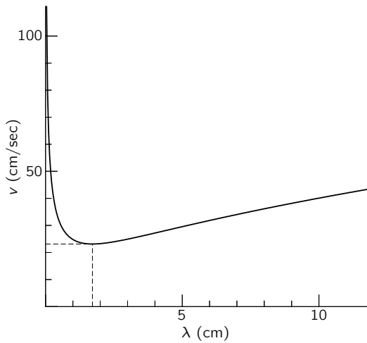
图 51.11: 水波的相速度对波长的曲线
