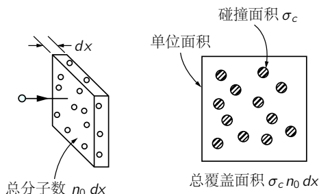
图 43.1: 碰撞截面
