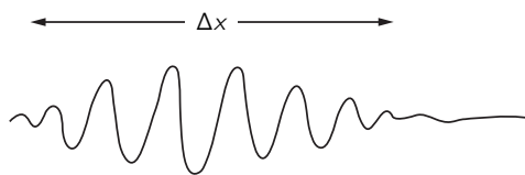
图 38.1: 长度为 \Delta x 的波包
