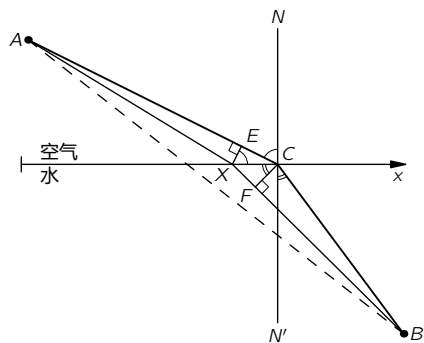
图 26.4: 费马原理对折射的说明
