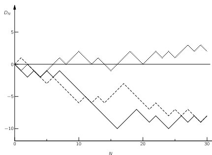
图 6.5: 无规行走取得的进度。横座标 N 表示所走的步数总数; 纵座标 D_N 表示离开起点的净距离
