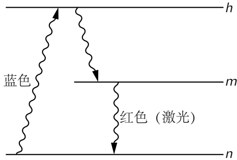
图 42.3: 如用蓝光将原子激发到较高的状态 h ，它可以发射一个光子使原子处于 m 态， m 态的原子足够多时就开始产生激光
