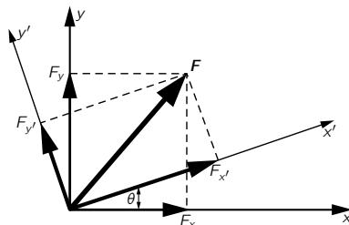
图 11.2: 角方位不同的两个坐标系 图 11.3: 在两个坐标系中力的分量
