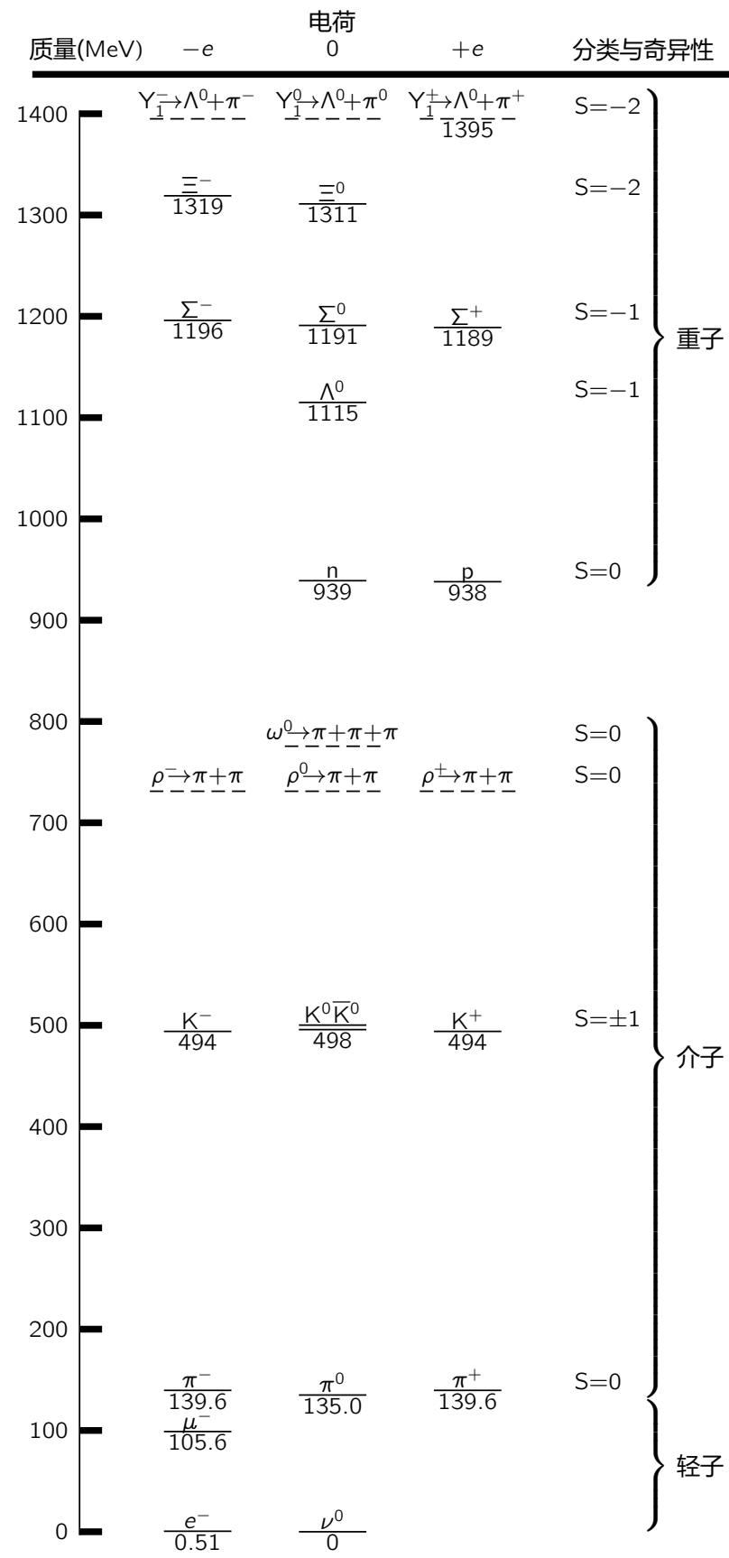
图 2.1: 基本粒子
