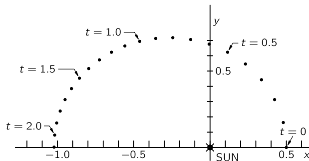
图 9.6: 由计算所得的行星绕日运动
