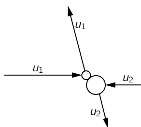
图 39.3: 从质心系来看两个不同分子间的碰撞
