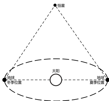
图 5.5: 利用地球轨道的直径作为基线, 可以用三角法测量靠近地球的恒星的距离 图 5.6: 靠近我们银河系中心的一个星团, 其中各恒星与地球的距离为 30,000 光年, 或约 3 \times 10^{20} 米
