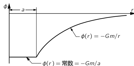
图 14.4: 由半径为 a 的球壳所引起的势能
