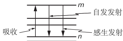
图 42.2: 原子内两个能级间的跃迁
