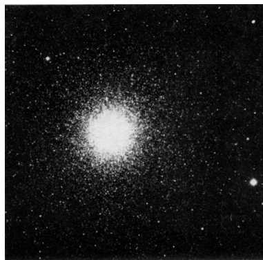
图 5.5: 利用地球轨道的直径作为基线, 可以用三角法测量靠近地球的恒星的距离 图 5.6: 靠近我们银河系中心的一个星团, 其中各恒星与地球的距离为 30,000 光年, 或约 3 \times 10^{20} 米
