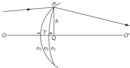
图 27.6: 两个曲率半径都为正的薄透镜
