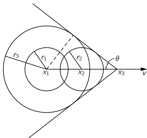
图 51.1: 冲击波的波前位于以源为顶点、半顶角 \theta = \sin^{-1}(c_w/v) 的锥面上
